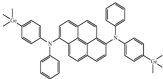
[D2]
