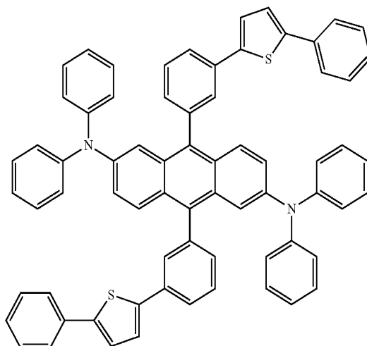
[B1]
